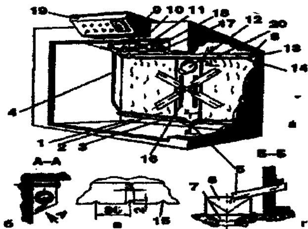
Рис.5. Модернизация выводного шкафа «Универсал-55»
