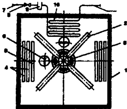
Рис. 3. Модернизация инкубационного шкафа «Универсал-50»
