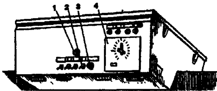
Рис. 1. Пульт управления инкубатора «Универсал-55»: 1 — световая сигнализация, 2 — тумблеры управления, 3 — предохранитель, 4 — регулятор температуры
