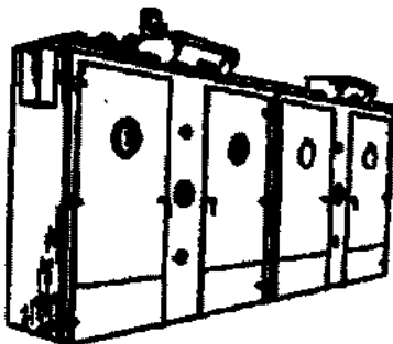
Рис. 2. Общий вид инкубатора ИКП-90
